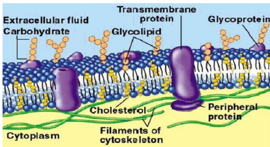
Gambar 1.1. Struktur Membran
