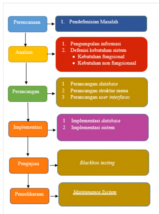
Gambar 3. 1 Metodologi Penelitian
