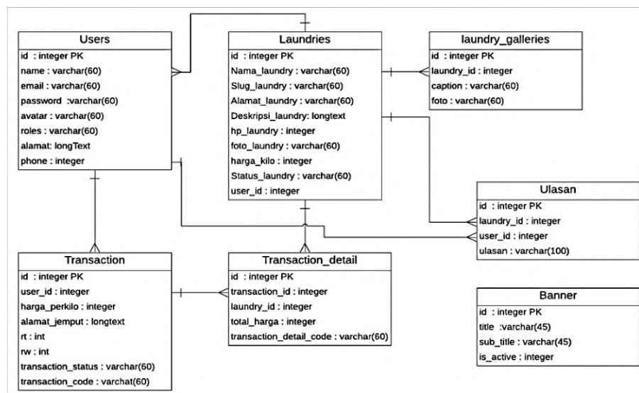
Gambar 4. 3 Perancangan Database
