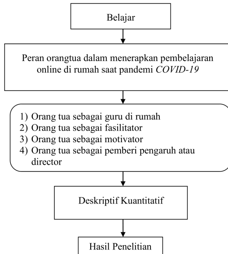
Gambar 1. Kerangka pemikiran
