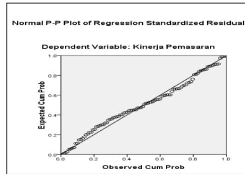
Gambar 2 Kurva Hasil Uji Normalitas
